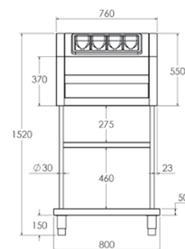
MEDIDAS DISPENSADOR
